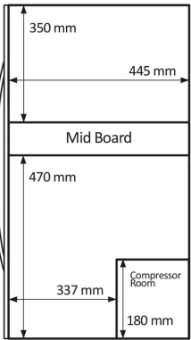
Width: 313 mm
